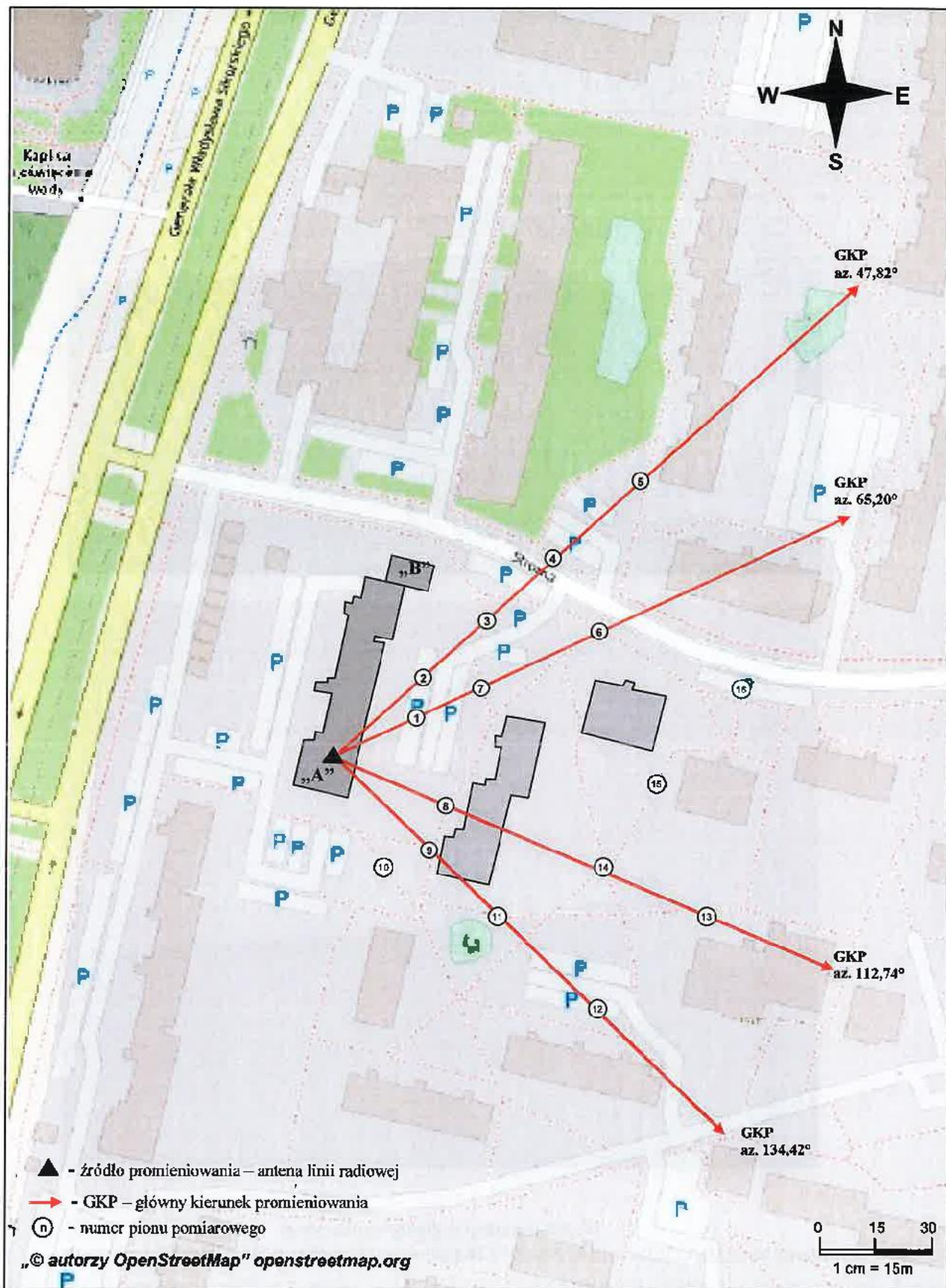
Rys. 1. Usytuowanie punktów i pionów pomiarowych w otoczeniu instalacji radiokomunikacyjnej Stacja Netia BIALB081-BIALM00057 Białystok, ul. Generała Władysława Sikorskiego 4
