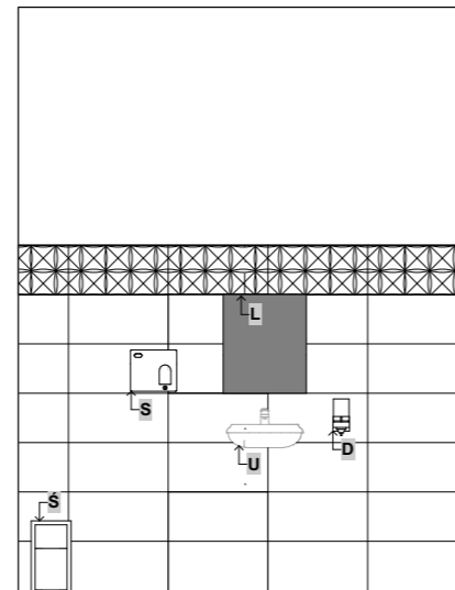
ROZWIĘCIE ŚCIANY B-B
