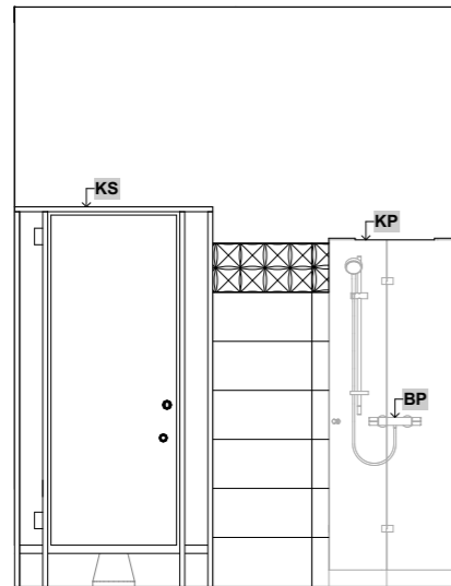
ROZWIĘCIE ŚCIANY A-A
