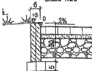
Szczegół "F" obrzeża 6x20cm skala 1:20
