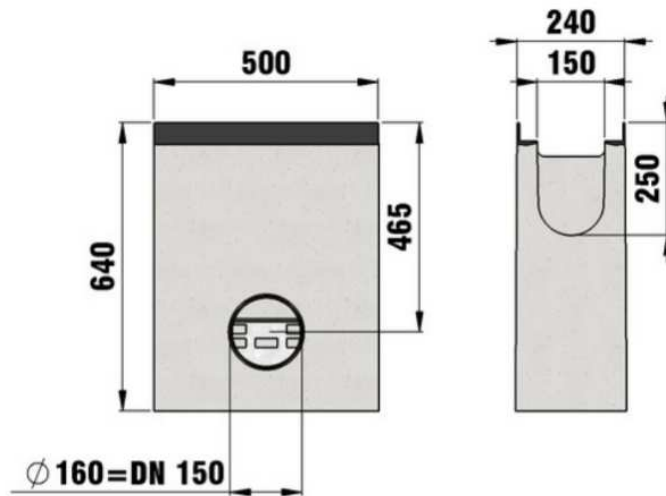
Studzienka z osadnikiem z tworzywa
