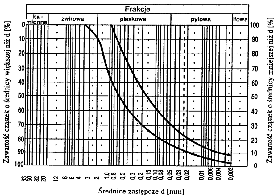
Tablica 2. Ramowy skład uziarnienia optymalnej mieszanki gliniasto-żwirowej
