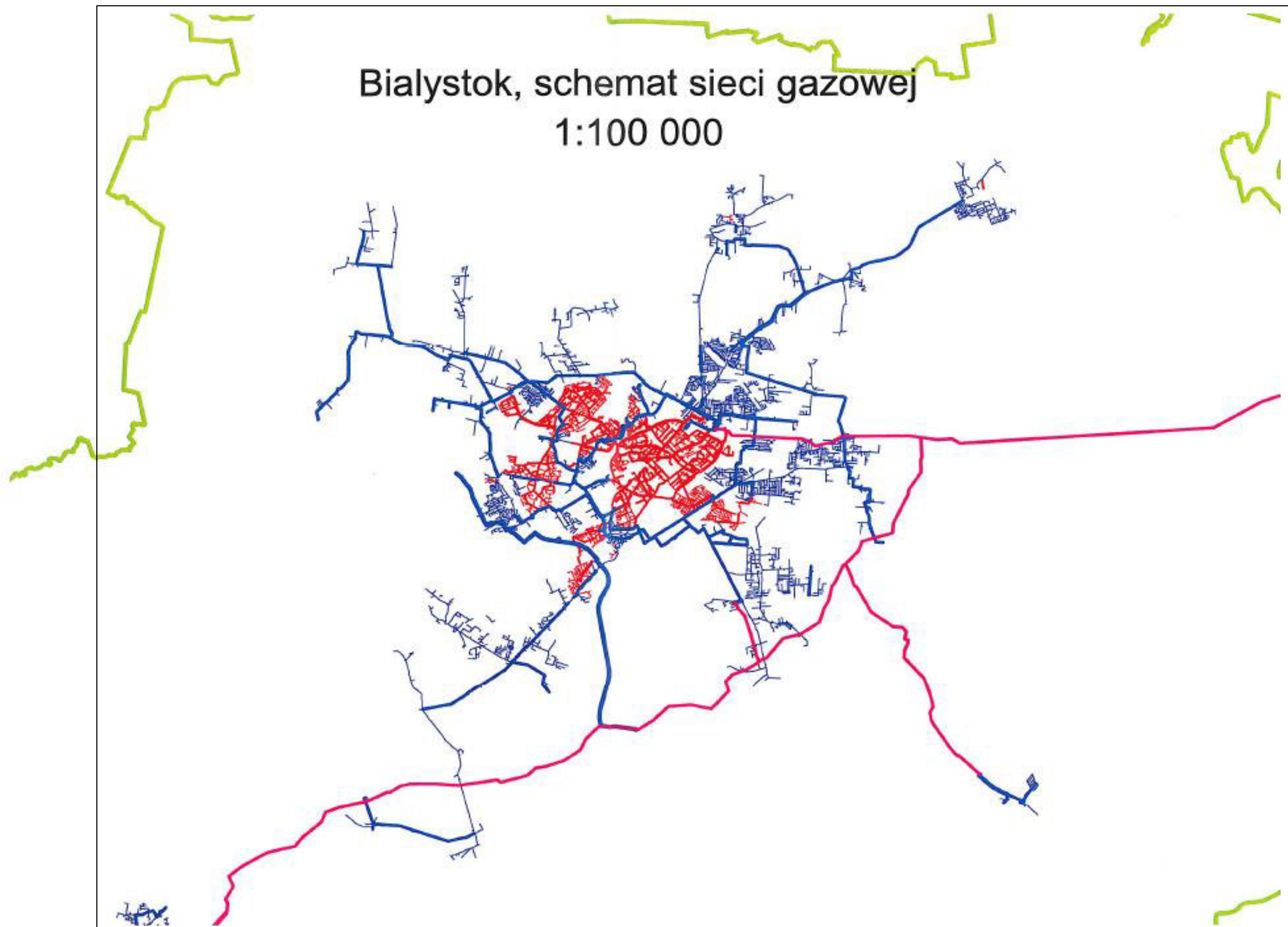
Rys. nr 12. Układ istniejących sieci gazowych na terenie Białegostoku
