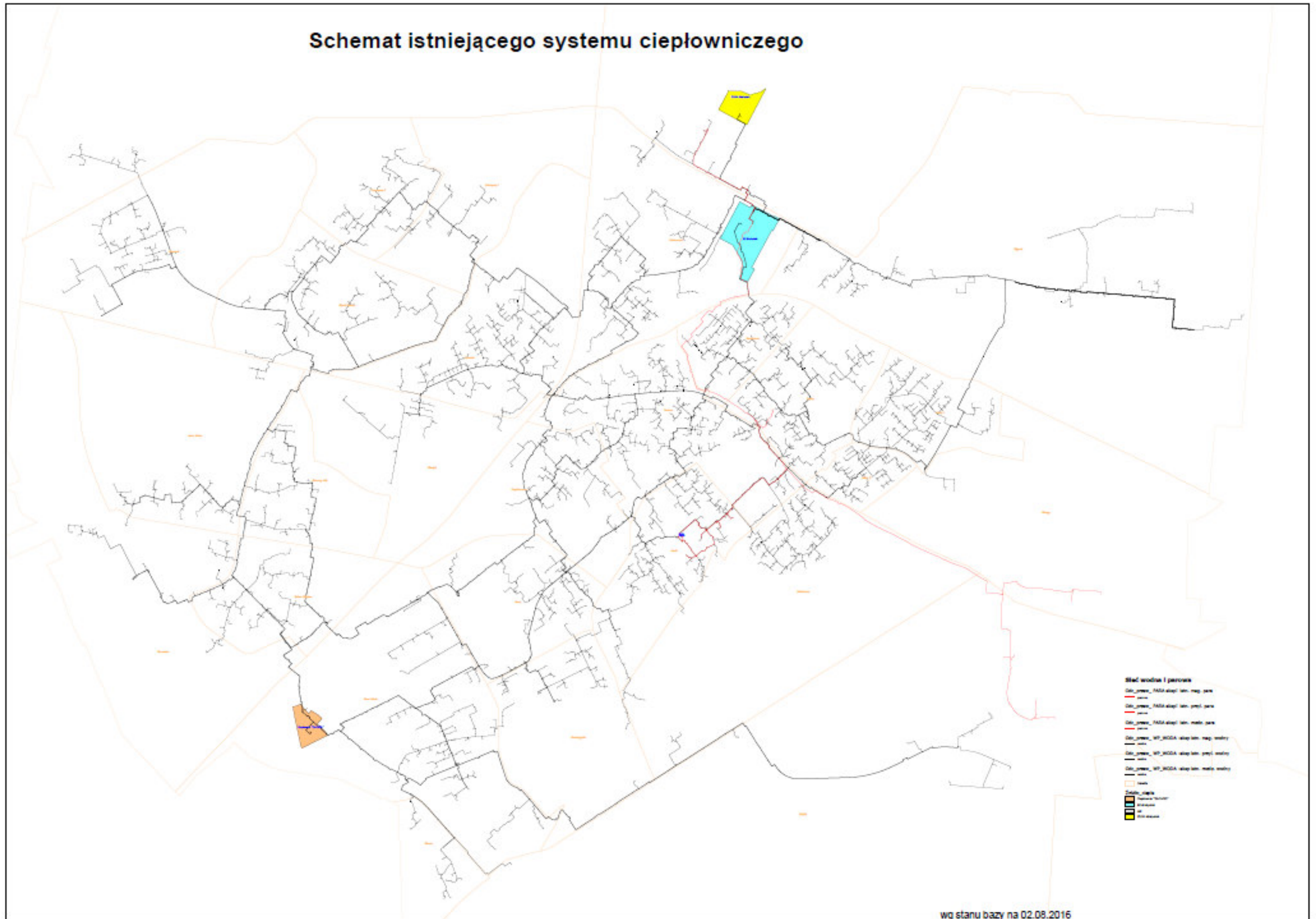
Rys. nr 6. Usytuowanie źródeł zasilania istniejącego systemu ciepłowniczego.
